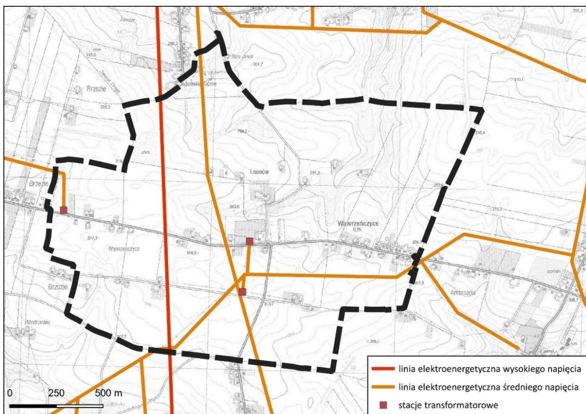
Rysunek 8. Przebieg linii elektroenergetycznych na terenie opracowania
